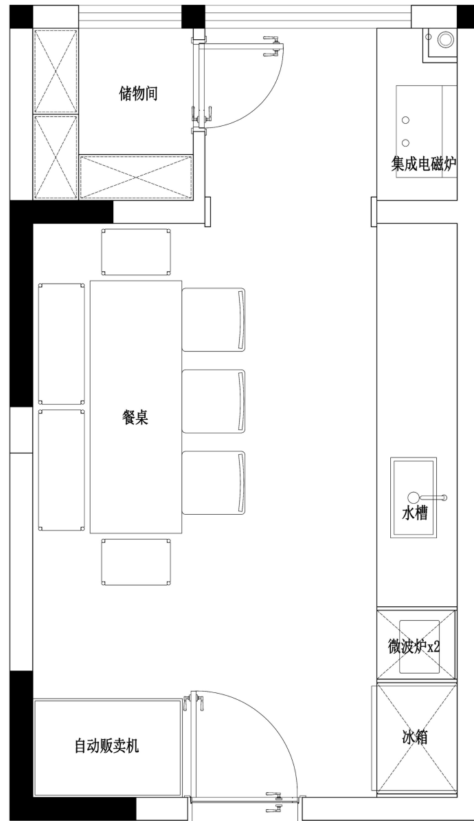
共享厨房平面图(方案一)
