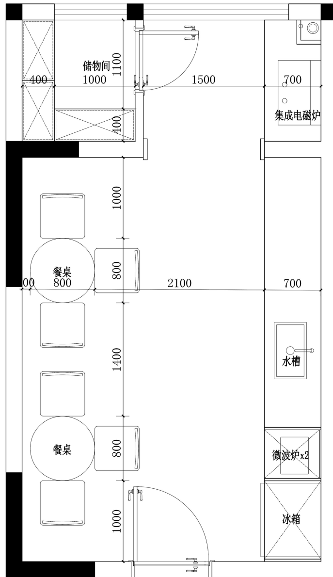
共享厨房平面尺寸图(方案二)
