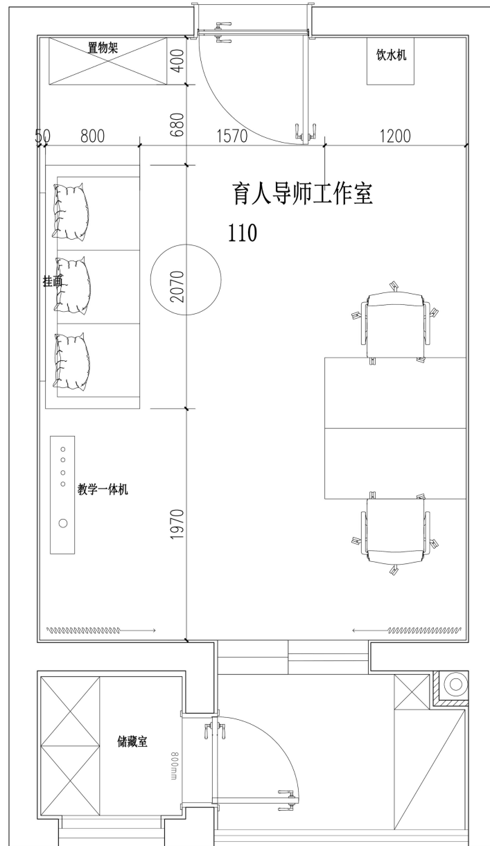
育人导师工作室平面尺寸图
