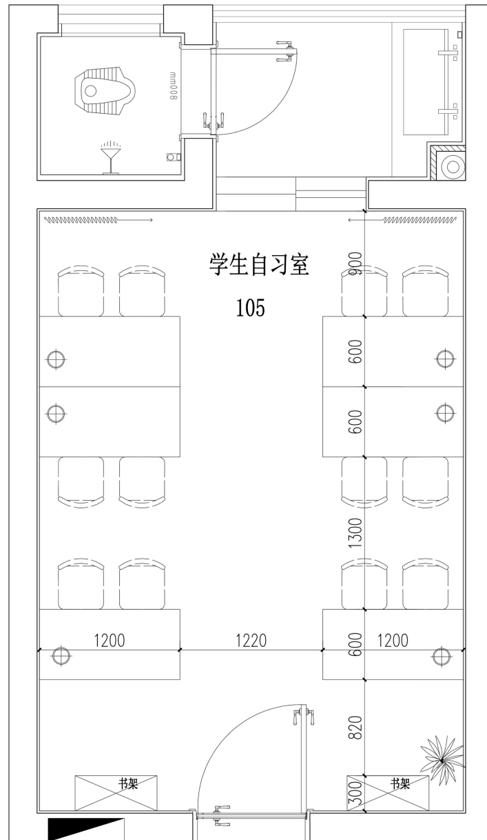
学生自习室平面尺寸图
