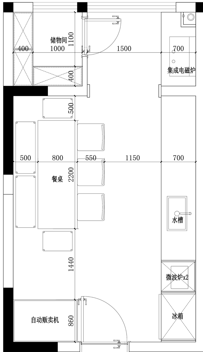
共享厨房平面尺寸图(方案一)
