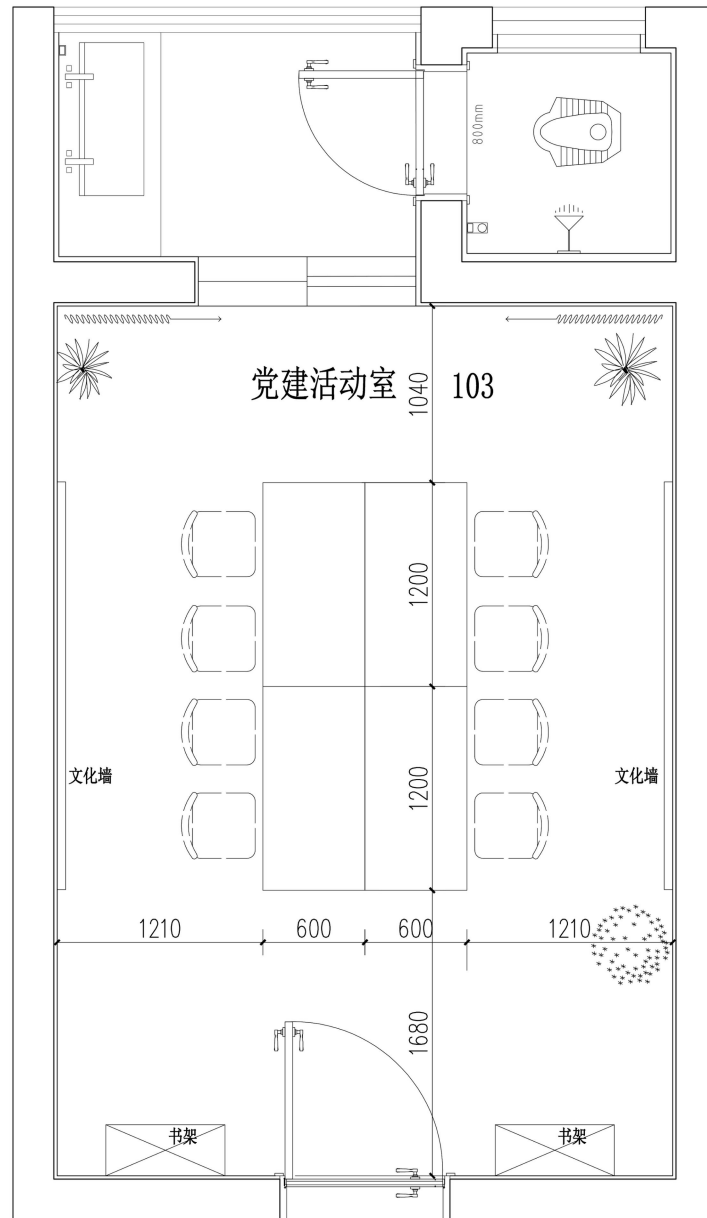
党建活动室平面尺寸图
