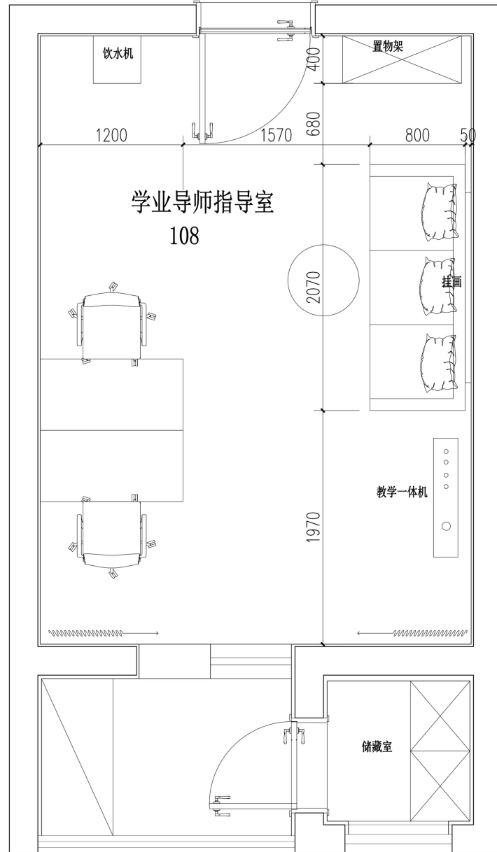
学业导师工作室平面尺寸图
