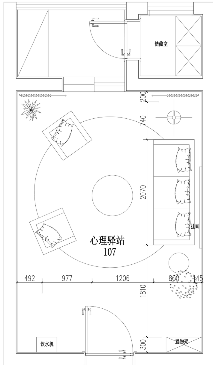
心理驿站平面尺寸图
